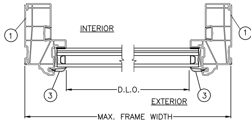
D 8 HORIZONTAL SECTION FRAME JAMB
